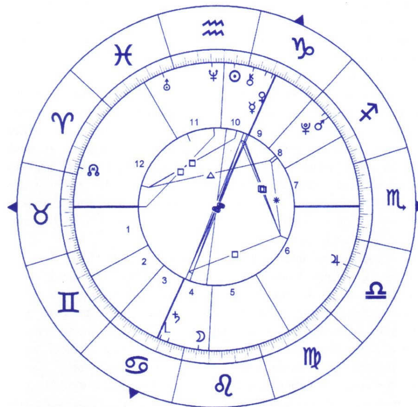
Aquarius Full Moon, 25th Jan. 2005, 11.32 h MET
